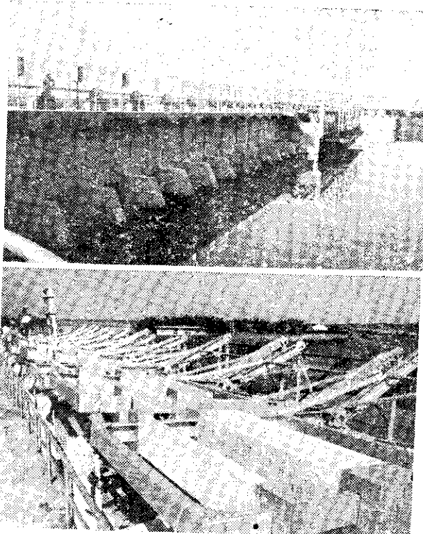
上：水利局建築宜五節湖防閘工程已完工。下：五節湖防閘式自動閘門。（袁統波攝）
