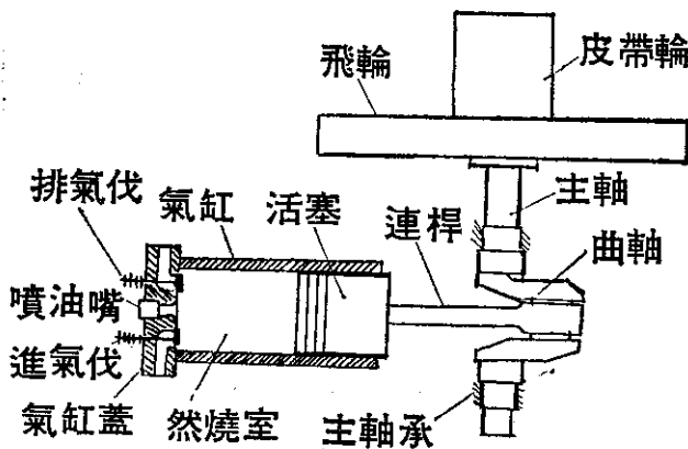
引擎動力產生部分構造
