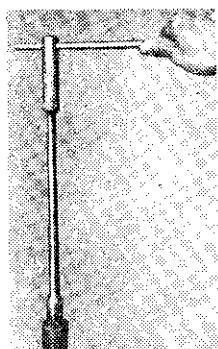
圖四 延長棒使用法
