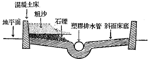
標準杆插用沙質苗床
