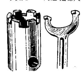
圖四 左：缺口套筒扳手 右：U型鉤形扳手
