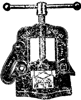
水管桌鉗
