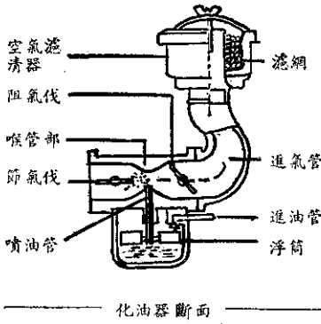
化油器斷面
