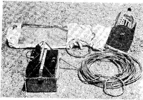
電動回轉式採茶機
