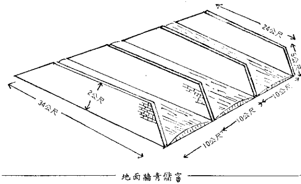
地面牆青儲窖
