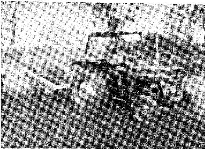
花生綜合收穫機：掘土部
