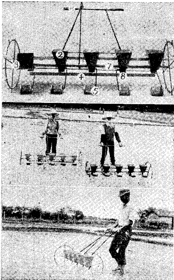
水稻直播機構造
