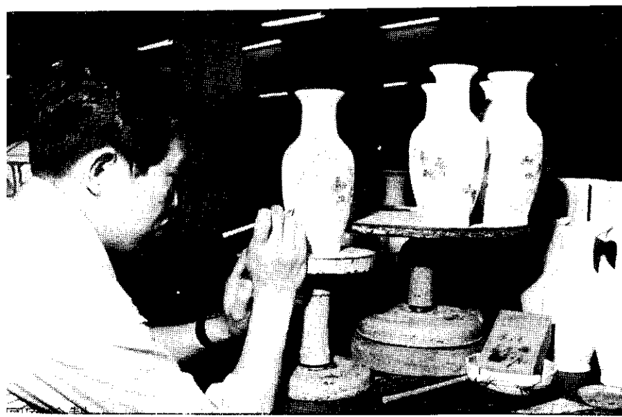
粗坯磨光
