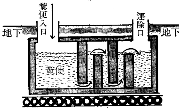
多隔式排糞槽
