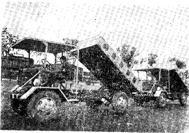
聯勤研製成功的農用車(張家寶)
