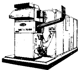
全自動烟葉兼用稻穀乾燥機
