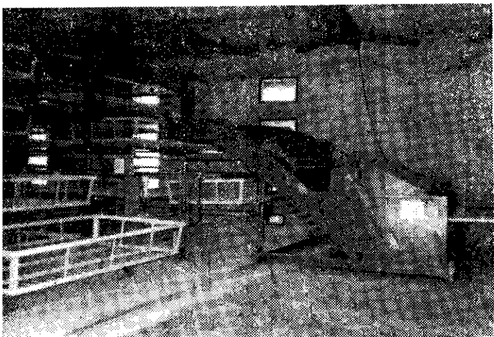
B-X壯蠶用多段循環式全自動飼育裝置
