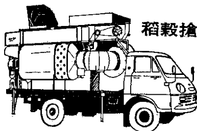
中型卡車型浮動層乾燥機
