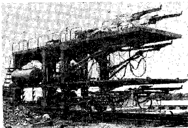
北平鐵路採用門型隧道開挖機 (中央社)
