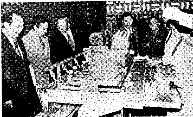
——農復會與養鵝協會舉辦的鵝蛋洗選機操作示範（中央社）——
