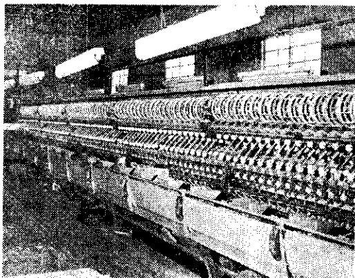
普通繅絲機
