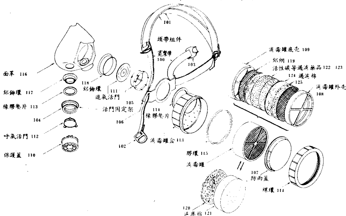
GM-300 防毒面具
