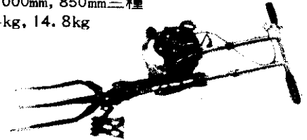
動力深耕機M-3型 ■引擎二衝程22.5cc. ■重量16kg ■深耕度約30cm
