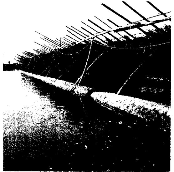
虱目魚越冬設備 (詹明宗 攝)
