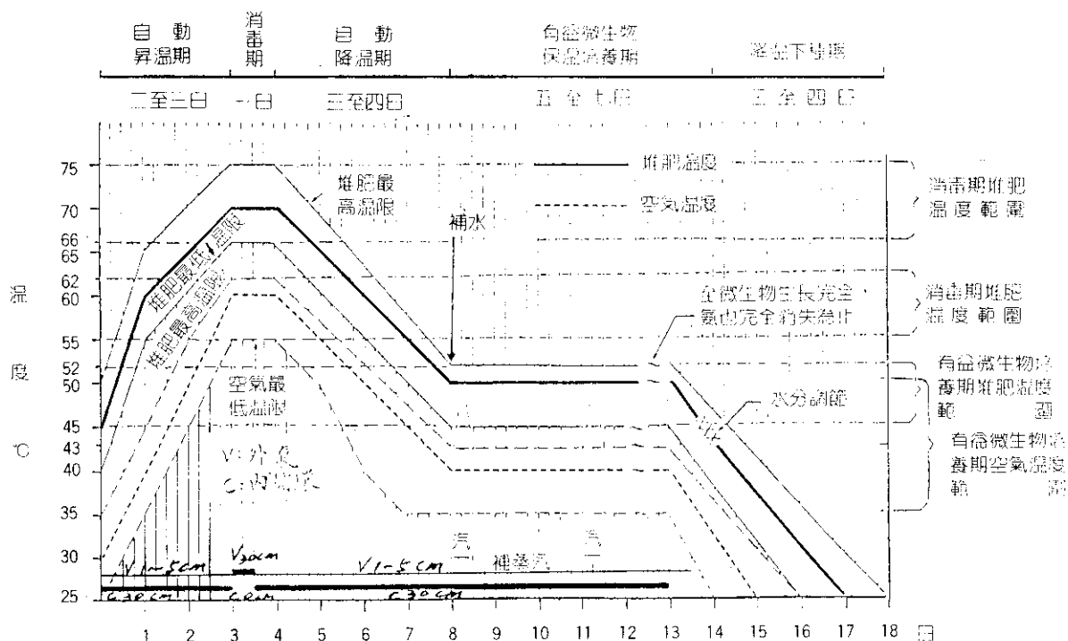
洋菇堆肥菌床發酵溫度預定曲線
