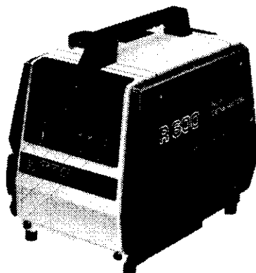
R600型 重量18.5KG 發電量600W R1200型 重量27.5KG 發電量1200W 使用4衝程電子點火引擎特別消音
