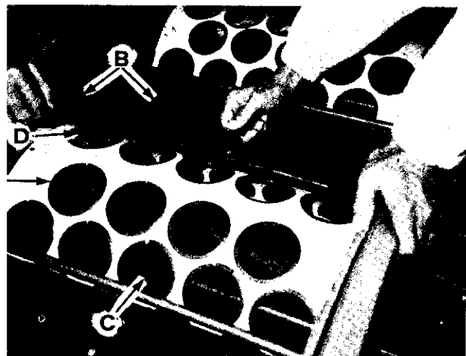
圖2. 改良之部位：(A)圓孔周邊；(B)平板及邊牆；(C)傳動木棍；(D)螺絲頭
