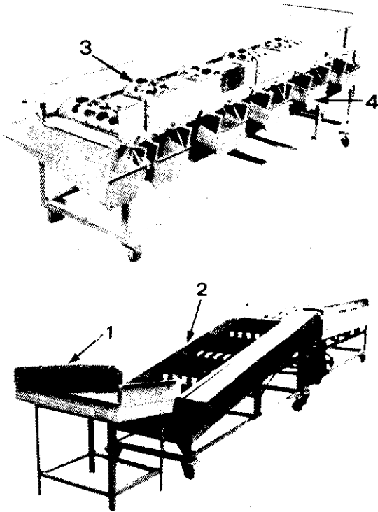
圖1. 未改良前之原型機①進料裝置②刷洗用輸送裝置③具有圓孔之選別滾筒④排果裝置
