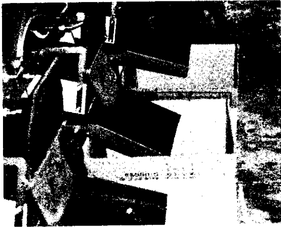
圖3. 排果出口處加裝彈簧式緩衝板
