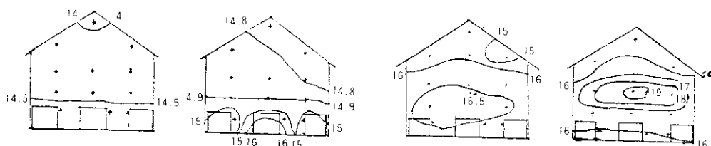
圖3. 冬季各種溫室狀況之溫度分佈例(清晨)
