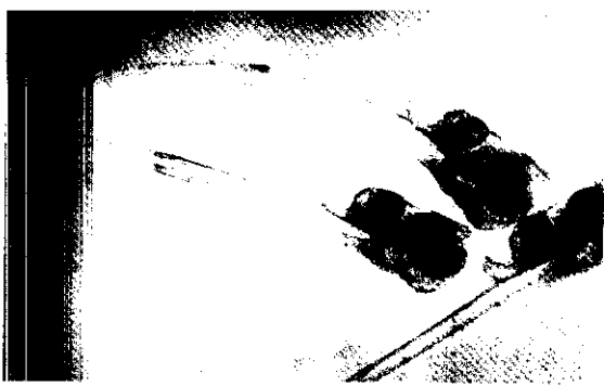
剛孵化：2天的泥鰍
