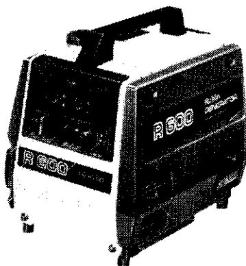
R600型 R1200型 重量18.5KG 重量27.5KG 發電量600W 發電量1200W 使用4衝程電子點火引擎特別消音
