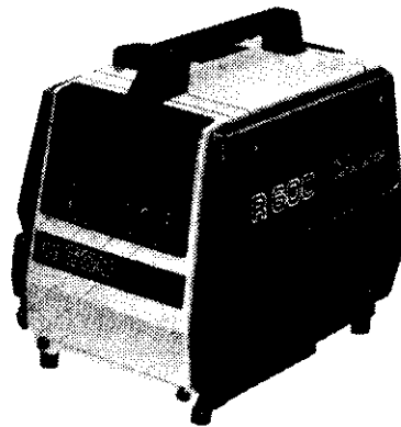
R650型 重量18.5KG 發電量600W R1200型 重量27.5KG 發電量1200W 使用4衝程電子點火引擎特別消音
