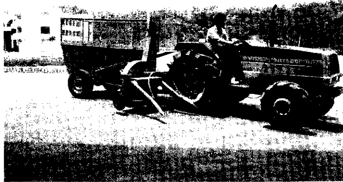
第二階段研究完成之旁載式狼尾草青割收穫機，已達80%作業功能要求。
