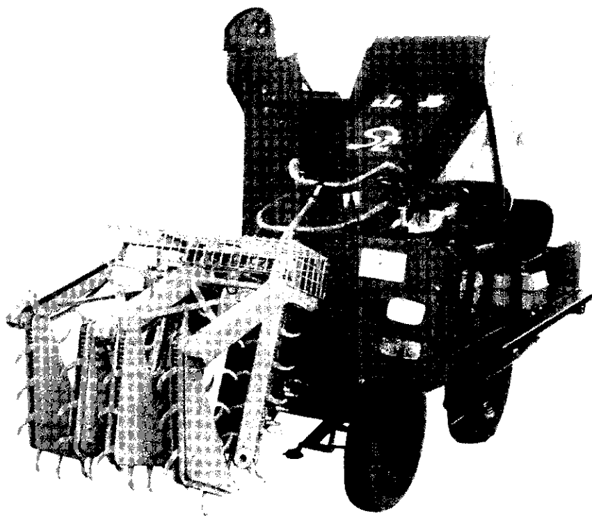
山能工業公司研製成功的花生收穫機
