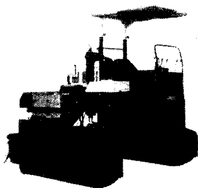
駕乘式施肥深耕車OMR-2型
