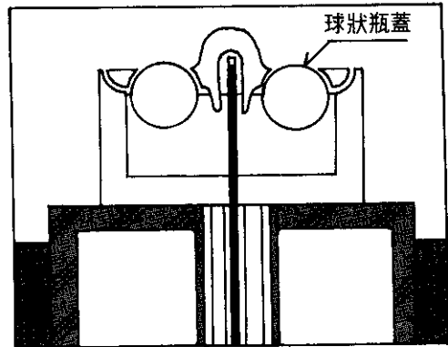
新型家畜飲水器的構造
