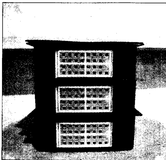
圖1. 九孔養殖籃每個高10公分、長60公分、寬40公分，圖為3個籃子的組合。
