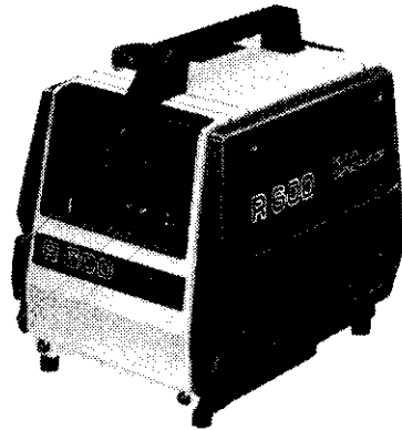
R650型 重量18.5KG 發電量650W R1210型 重量27.5KG 發電量1200W 使用4行程電子點火引擎特別消音
