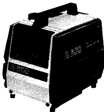
R650型 R1210型 重量18.5KG 重量27.5KG 發電量650W 發電量1200W 使用4行程電子點火引擎特別消音
