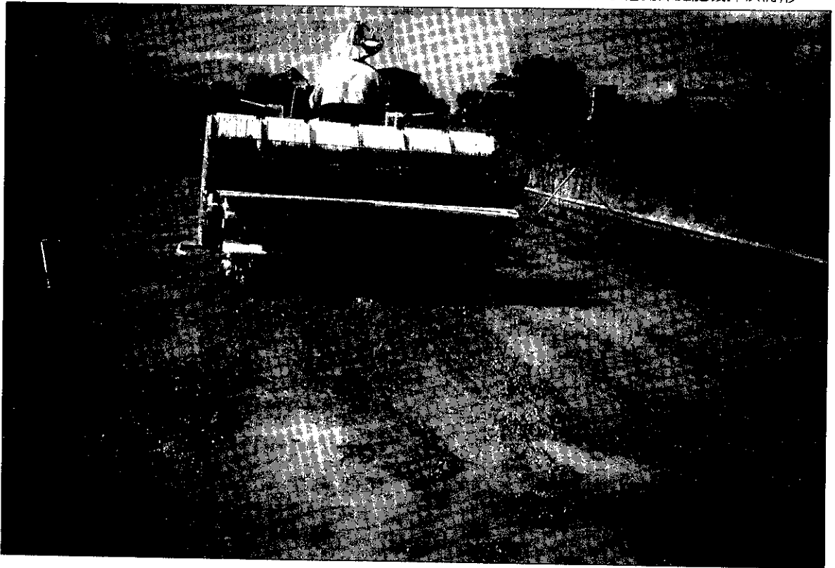
圖為竹北鄉農友楊金土操作水稻側條施肥機插秧情形
