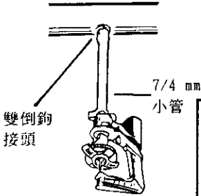
壓入型 系統
