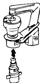
防蟲罩的組裝法
