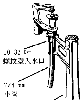
鑰入型 小支柱
