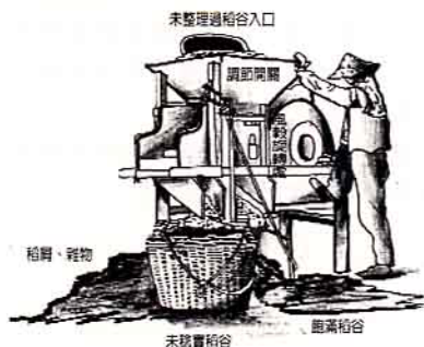
傳統農村風穀機各部結構簡圖
