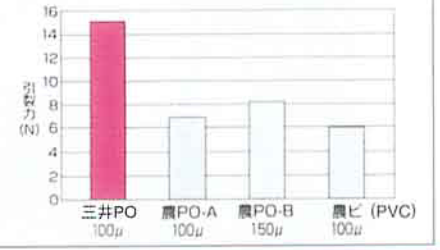
●エルメントルフ引裂力(MD)
