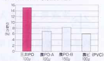
●エルメンドルフ引裂力(MD)
