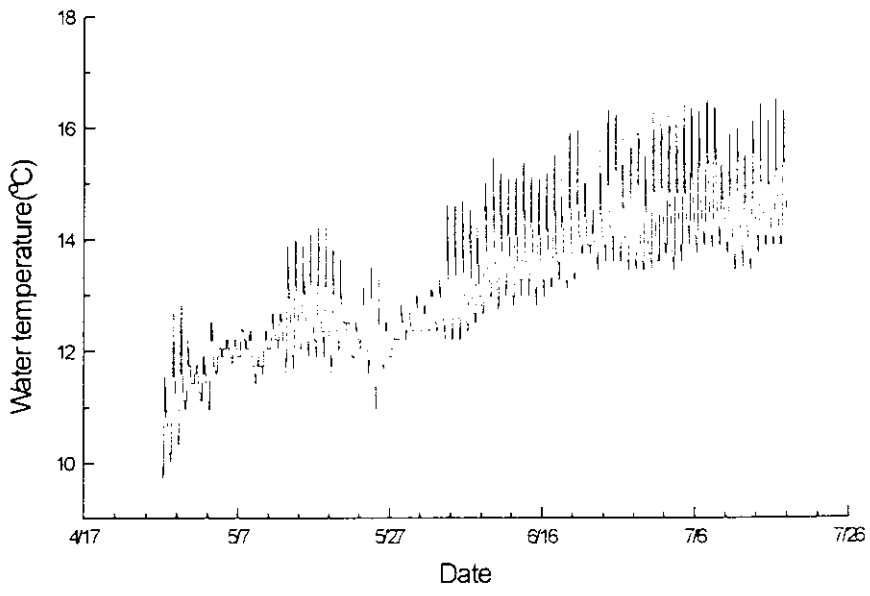
圖十一：三號壩上春夏季水溫變化圖（1996.4.27--1996.7.17）
