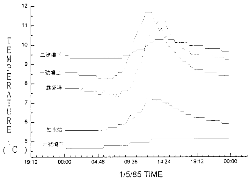
圖六：七家灣溪各河段冬季水溫變化圖：包括七家灣溪上游（六號壩下）、中游（抽水站、二號壩下）以及下游河段（一號壩上與露營場）各點的96年1月5日水溫比較圖。
