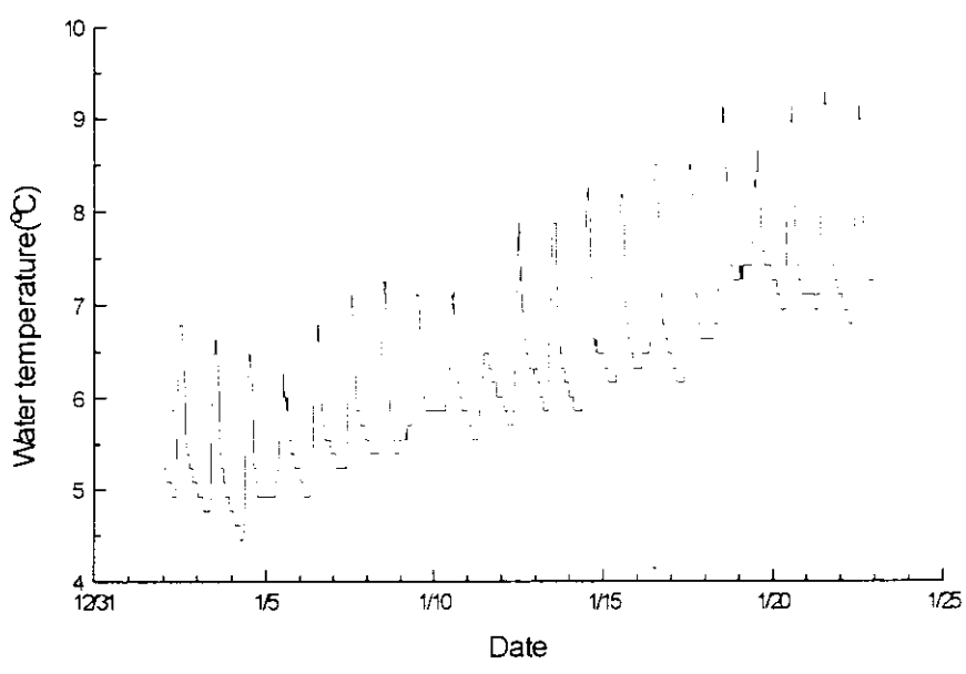
圖十：三號壩上冬季水溫變化圖（1996.1.2--1996.1.22）
