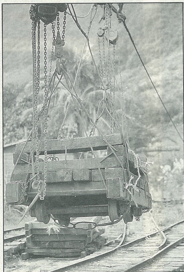
索道台車
