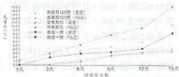
圖7 高雄2號與屏東長茄於不同儲藏環境下失重率變化
