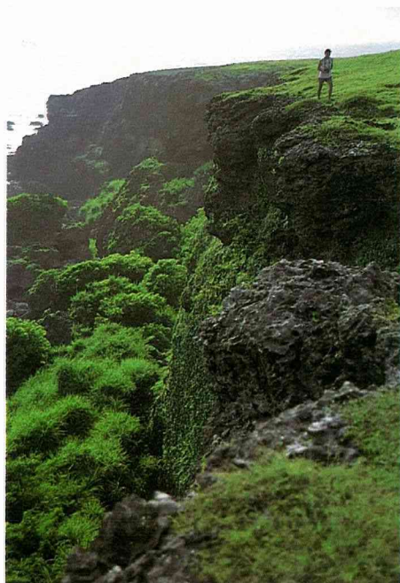
受劇烈海蝕作用造成的 崩崖地形
