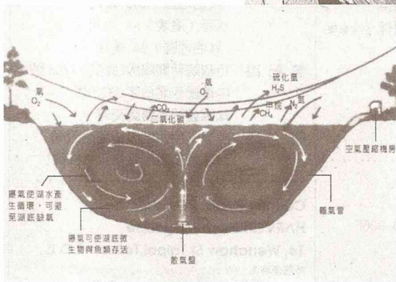
■澄清湖、鳳山水庫曝氣工程示意圖。
