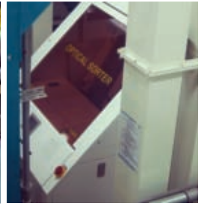
「瀑布式色彩選別機」可精準地去除白米中的壞米粒和雜質
