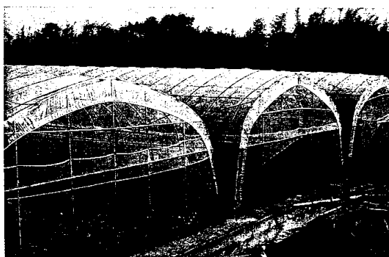
圖2：設施間可挖溝灌水
